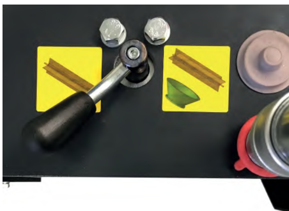
Páka zapínání hlavního/bočního kartáče
